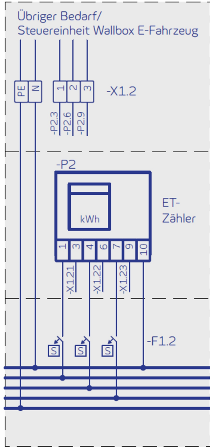
Zählerschrank Haushalt
