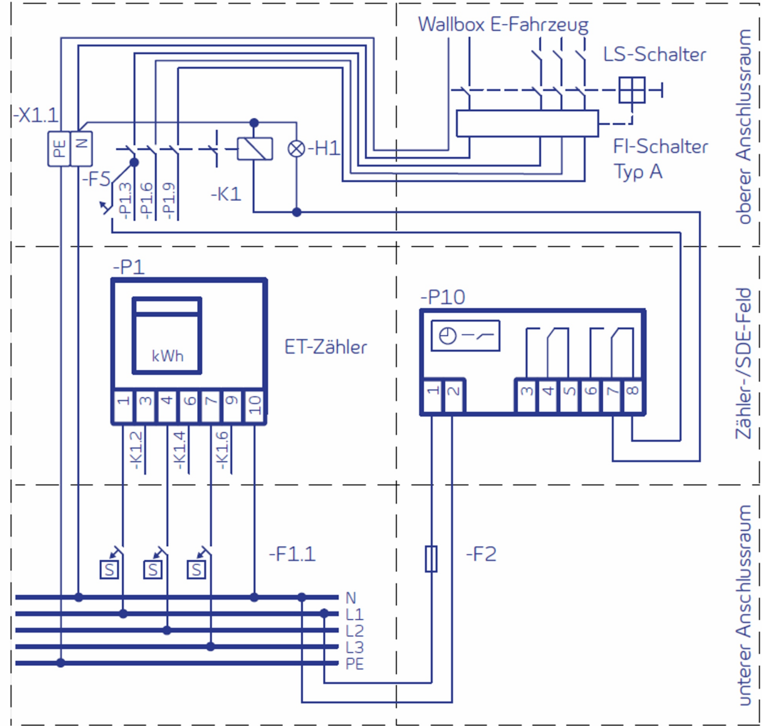
Zählerschrank für Wallbox (gemäß §14a EnWG)
