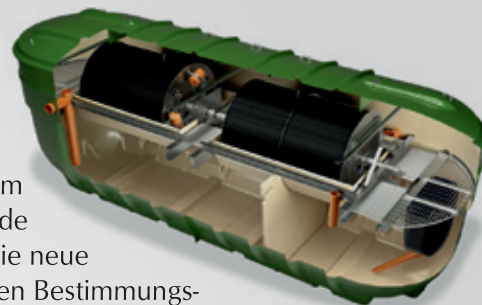
Blick in das Innere einer Kleinkläranlage am Modell. Foto: www.kingspan.com
